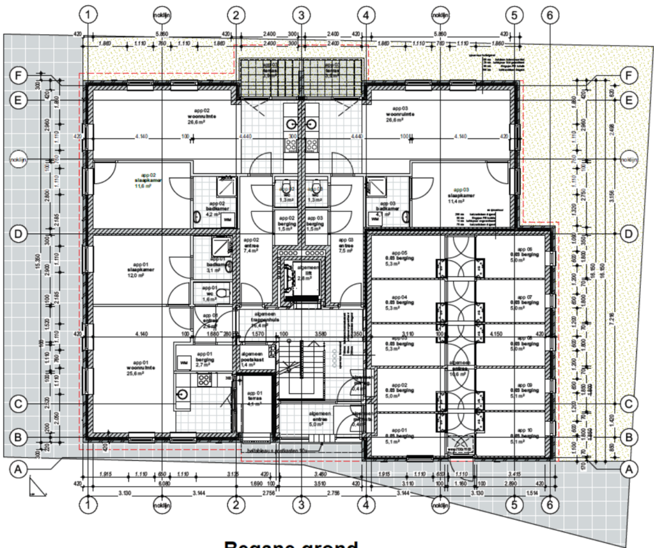
Begane grond
